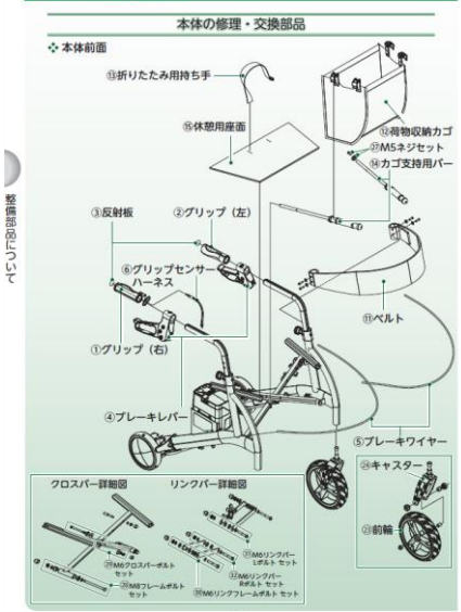
(出所) ロボットアシストウォーカー-RT.2 (RT.ワークス株) 「整備マニュアル」より抜粋
